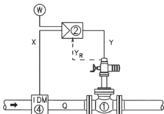
Регулирование потока: постоянный расход (Q)
