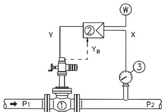
Регулирование давления: Постоянное выходное давление (P2)
