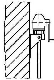
Стенной кронштейн
